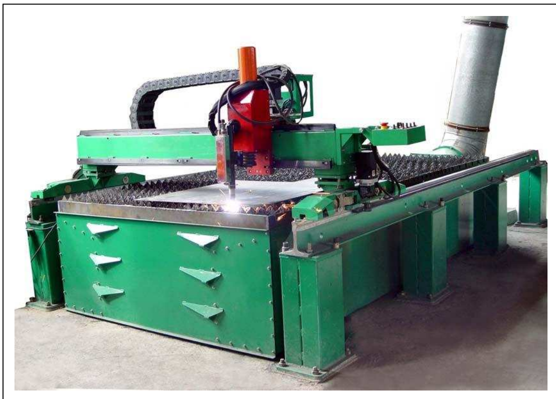
Машина высокоточной скоростной плазменной резки «Метеор»
