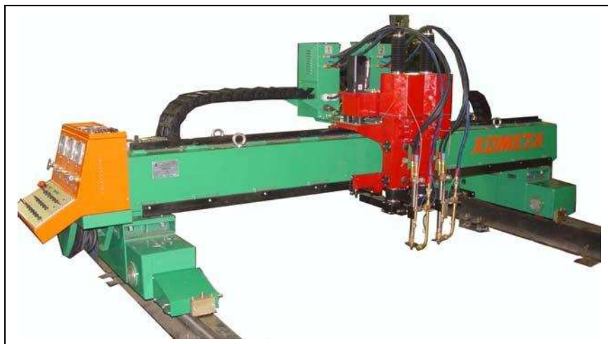
Машина «Комета-2М» с кислородной оснасткой
